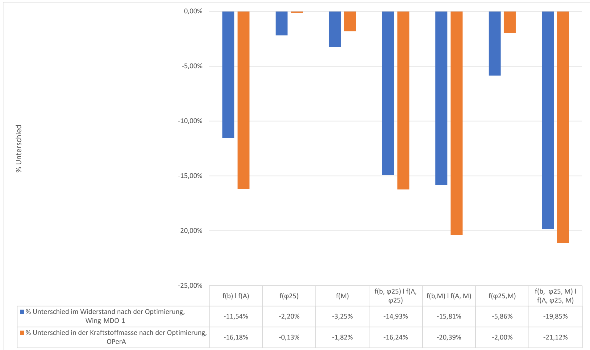
Bild 6.1 Prozentuale Unterschiede im Widerstand und in der Kraftstoffmasse nach der Optimierung mit Wing-MDO-1 und OPerA
